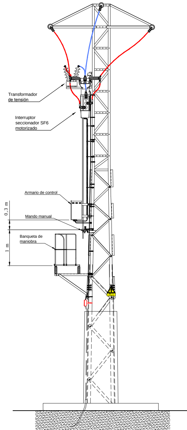
VISTA LATERAL
