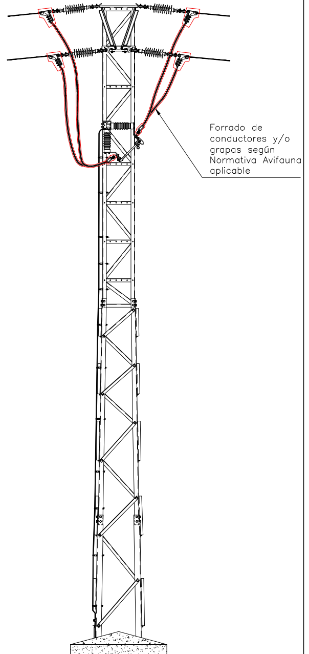
VISTA LATERAL
