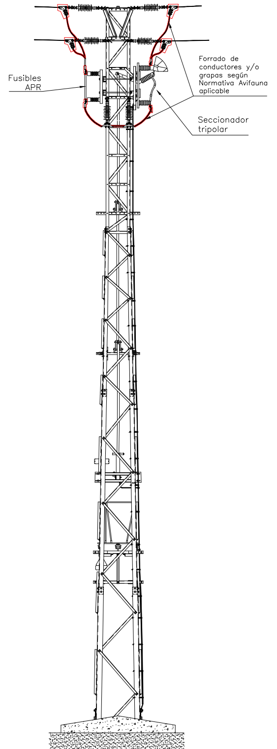
VISTA LATERAL
