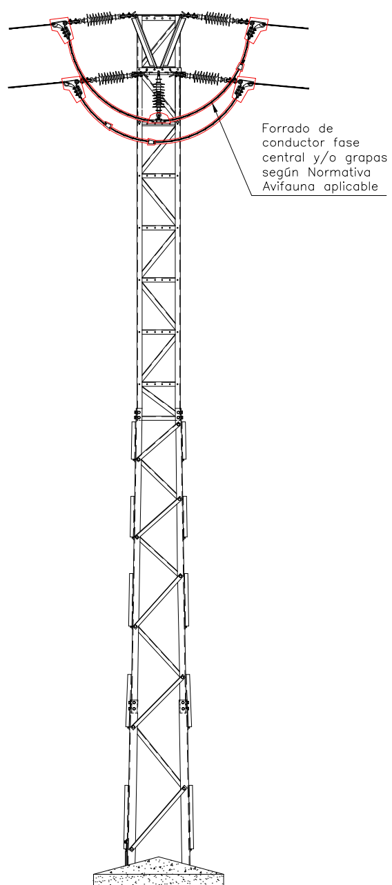
VISTA LATERAL
