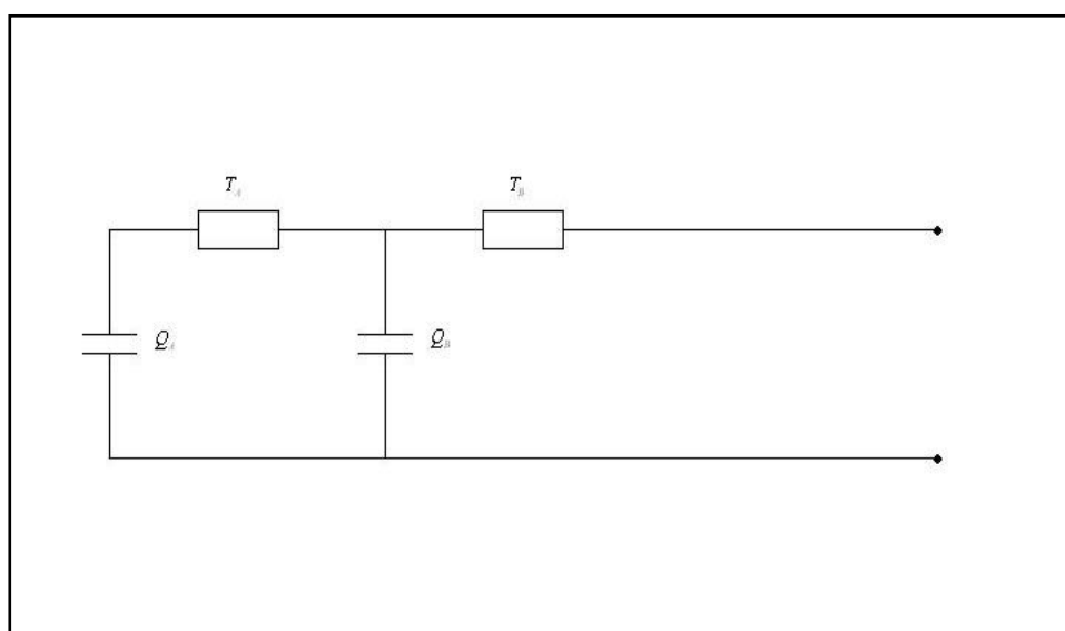
Figura 16: Red equivalente al cable para los cálculos de la respuesta transitoria
