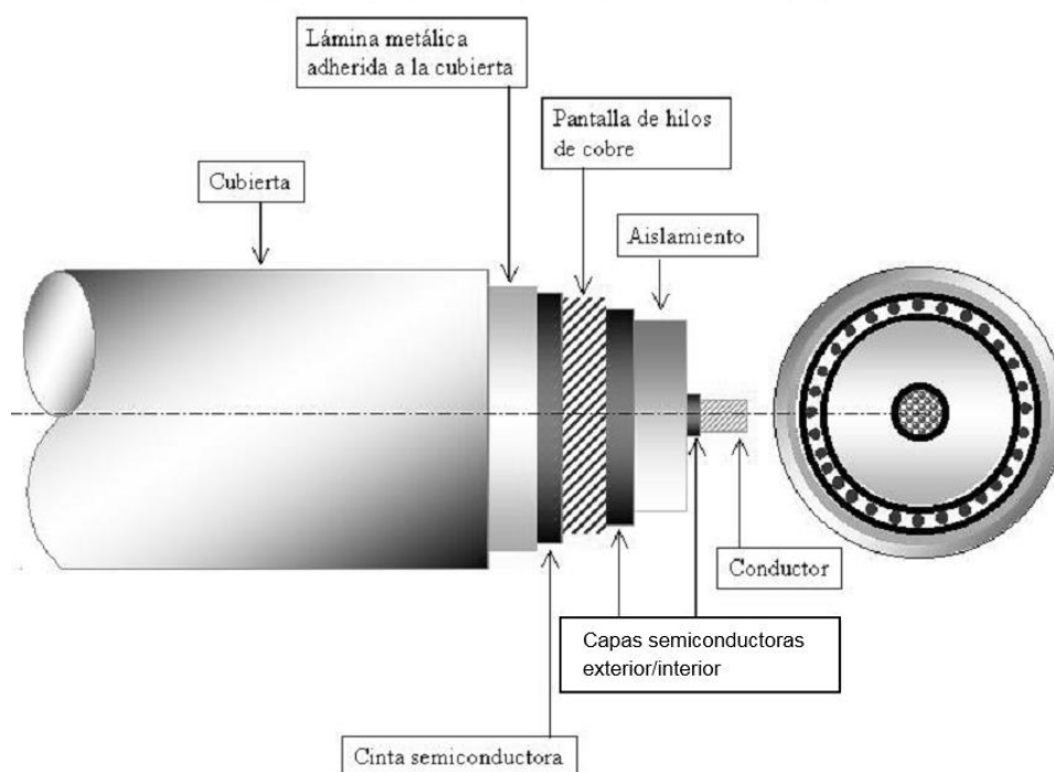
Figura 1: Constitución de los cables subterráneos
