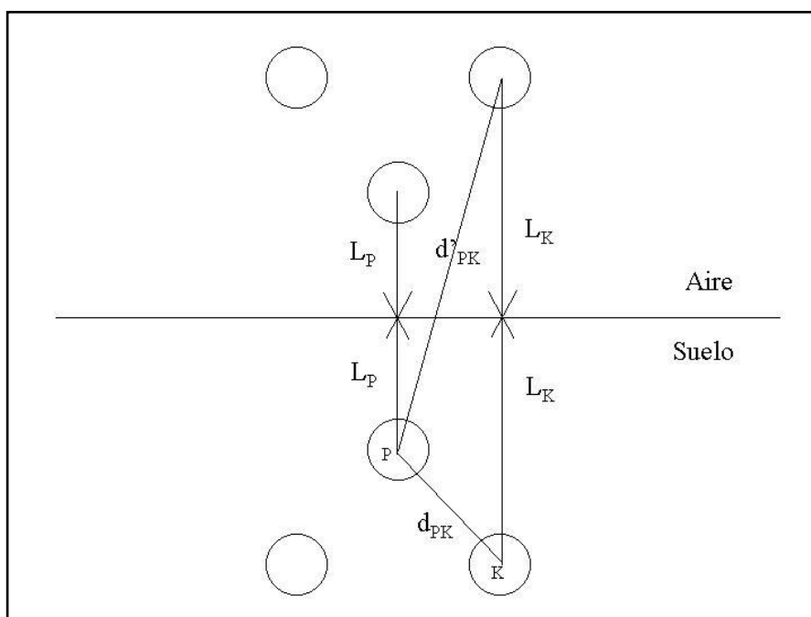
Figura 14: Diagrama que muestra un grupo de cables y sus imágenes con relación a la superficie aire-suelo.
