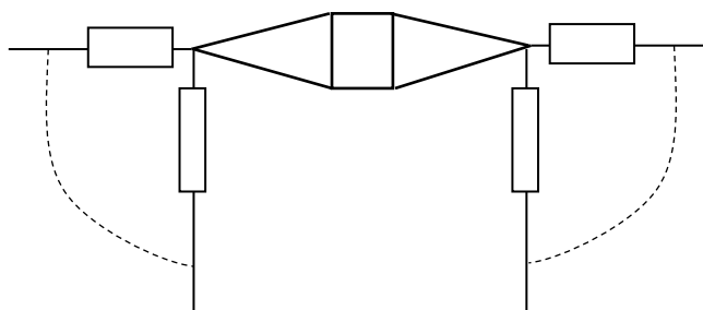
Fig 1 Esquema entronque en línea simple circuito
