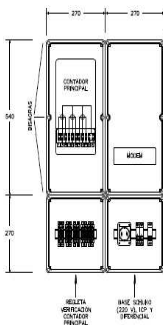
Figura 3. Conjunto modular
