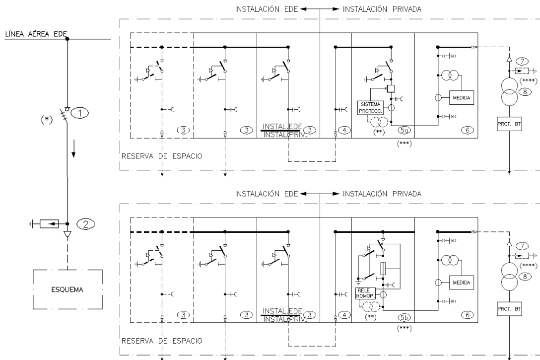
TIPO ACOMETIDA 2
