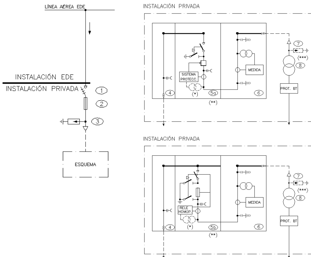
TIPO ACOMETIDA 1
