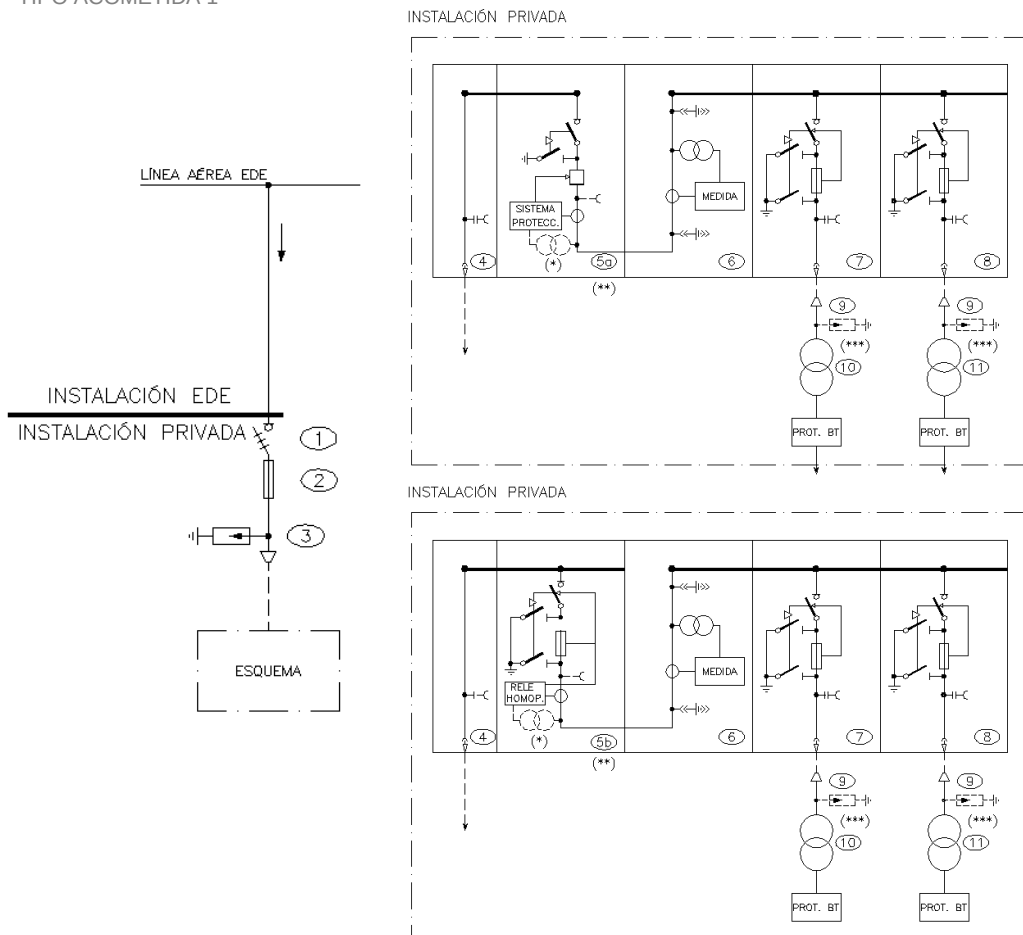
TIPO ACOMETIDA 1
