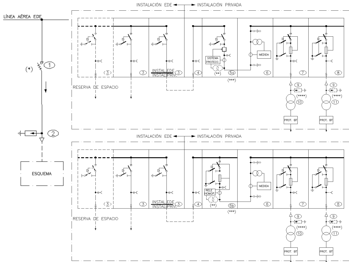
TIPO ACOMETIDA 2
